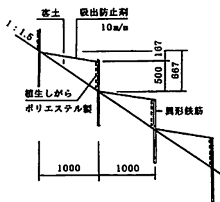
図-1 階段状植栽床
